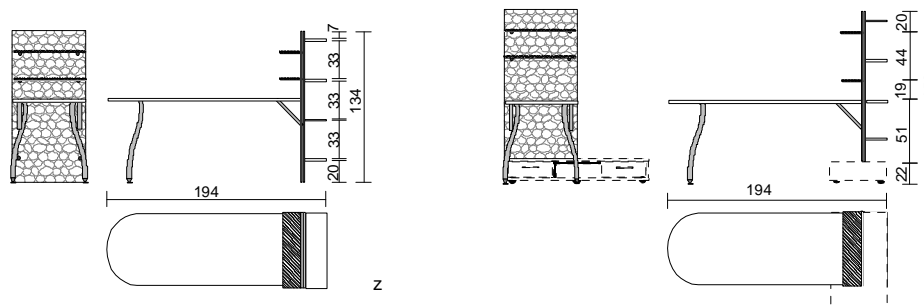
Bild 1 (Variante bodenstehend)
