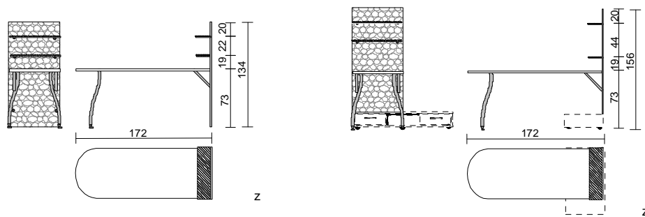
Bild 1 (Variante bodenstehend)
